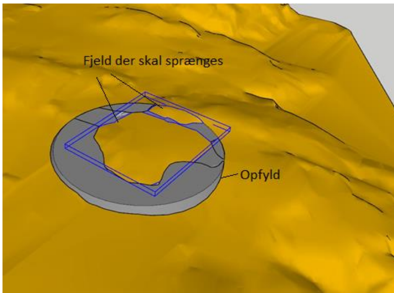
Billede 1: Hindringer ved helikopterflyveplads og ved ind- og udflyvningsflade
